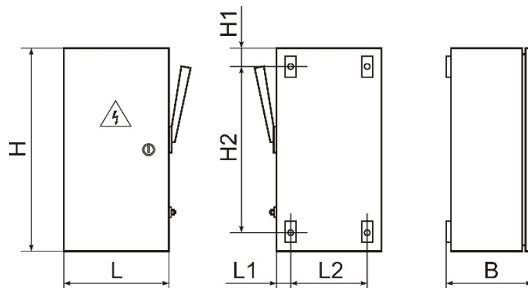
Общий вид и габаритные размеры ящиков силовых ЯРП11М-3
